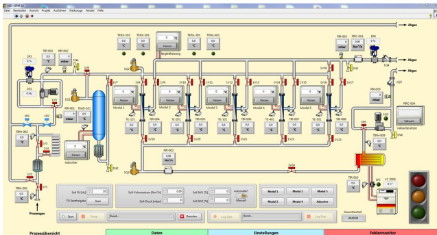
Fließschema einer mehrstufigen automatisierten Gaspermeationsanlage.
